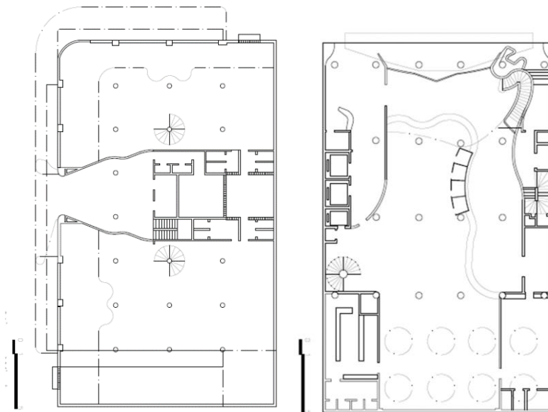
Figura 20: Edifício Caramuru
